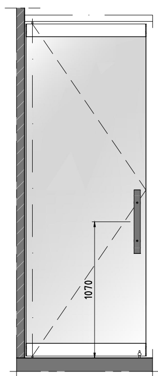
Communicatiepaneel
