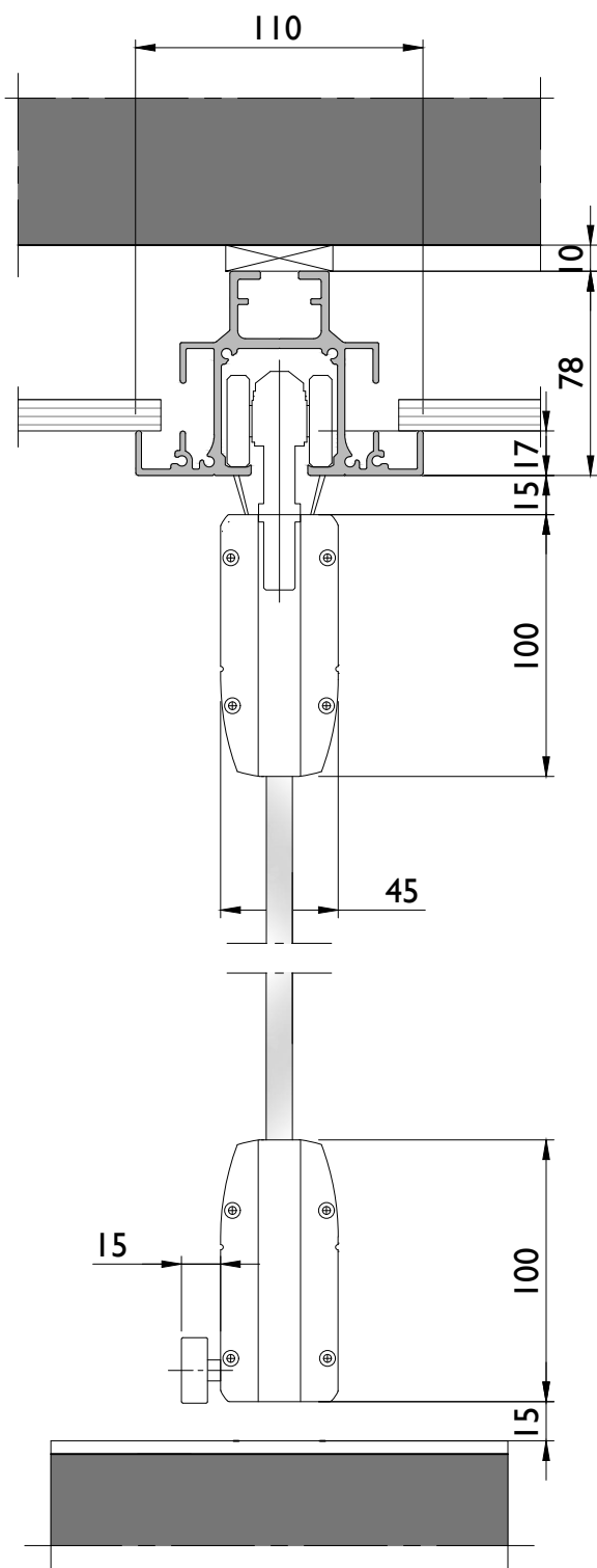
I-punts ophanging
