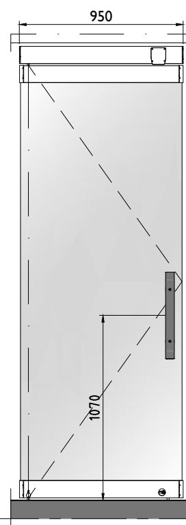
Deurpaneel
