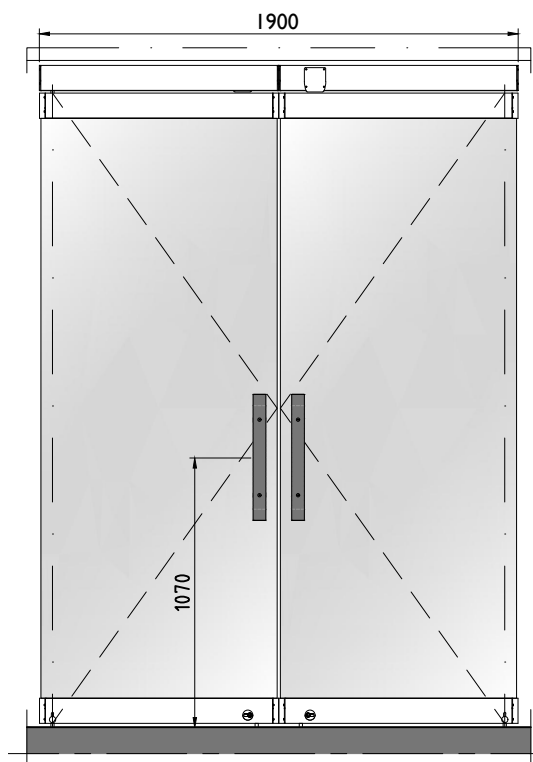
Dubbel deurpaneel met Standaard deurgreep
