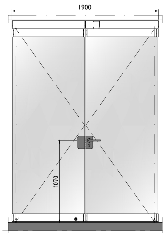
Dubbel deurpaneel met Slotkast tegen slotkast met kruk
